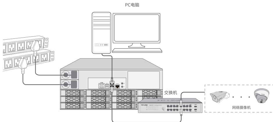
图3-4 NVS连接示意图
