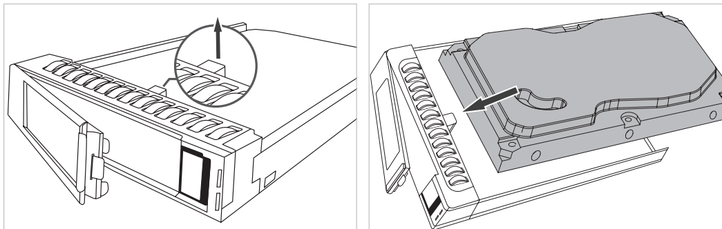
图3-3 安装硬盘
